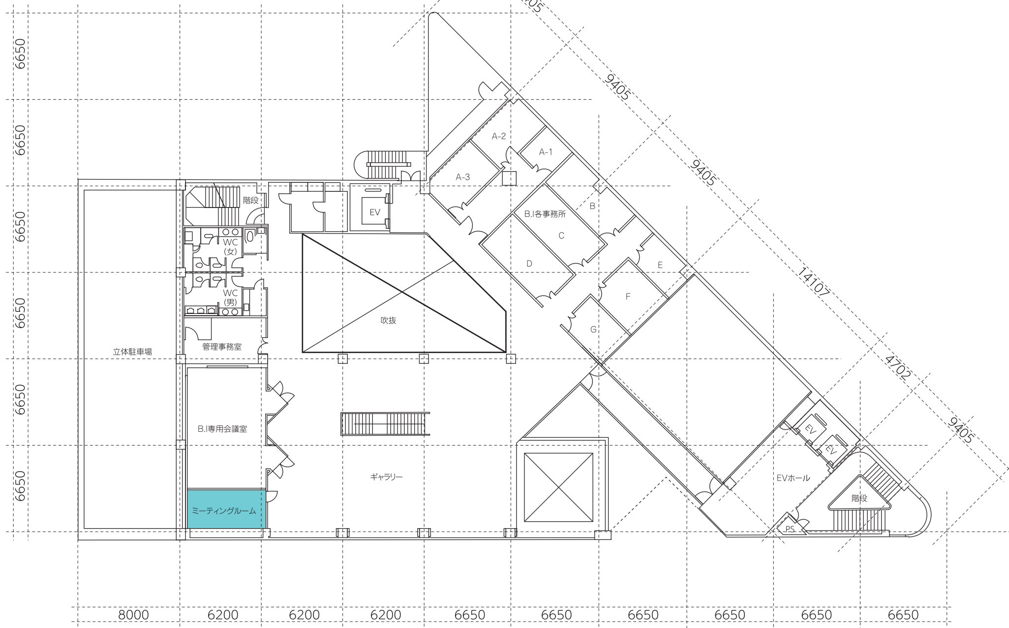
多治見市産業文化センター 2階平面図(単位はmm)
